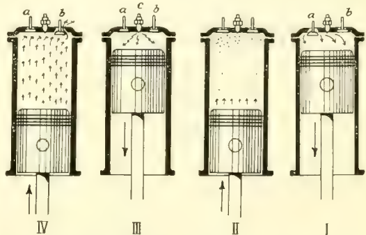
סכעמאַטישע פאַרשטעלונג פון די 4 טאַקטן אין אַ צילינדער:
